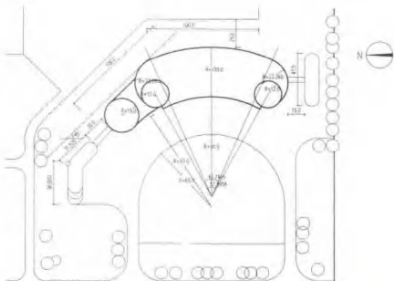
总平面
