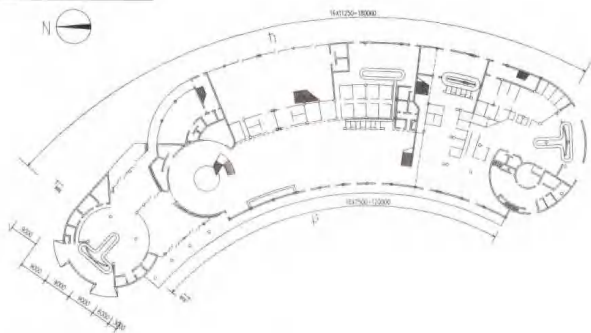
首层平面
