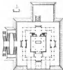
平面
