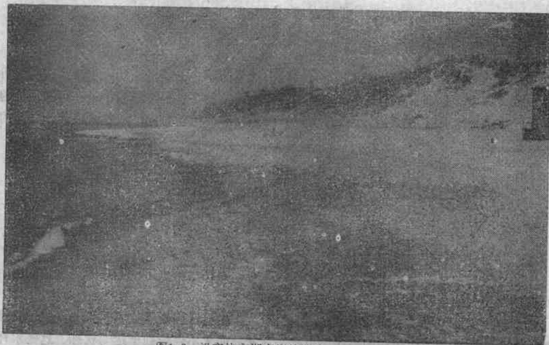
图1-2 沿密执安湖南岸的沙丘
