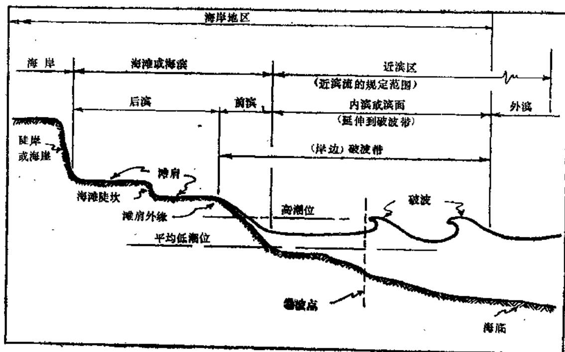
图1-1 海滩剖面及有关的术语
