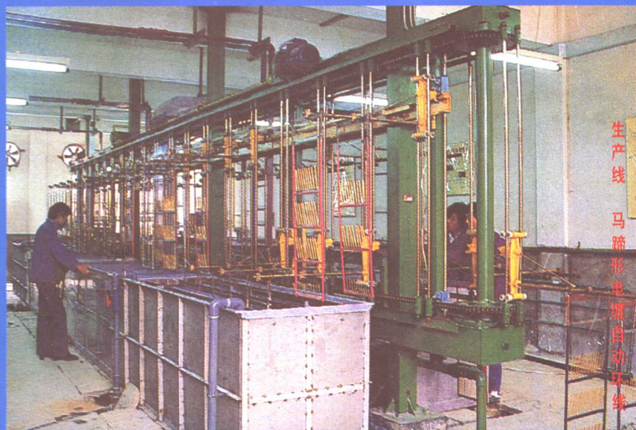
生产线（专用自动车床 加工天线零件）
