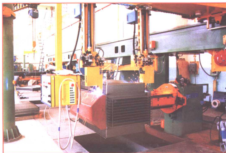
引进：联邦德国制造的变压器波纹油箱成型生产线
