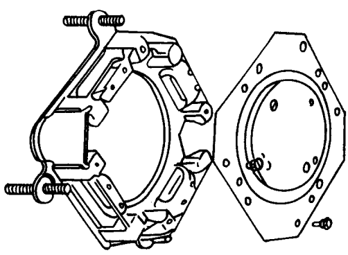
单线槽分线盒装配示意图
