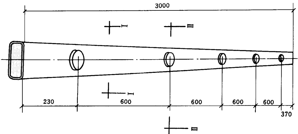
地面金属线槽外形尺寸图
