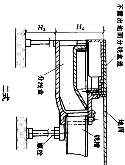
分线盒安装示意图
