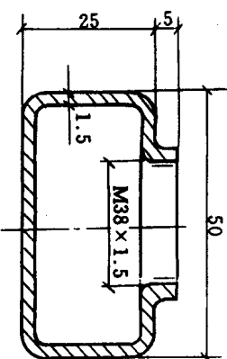
II - II (50 系列)
