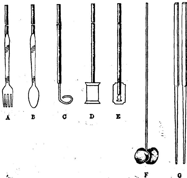
图 1 瓶型操作工具
