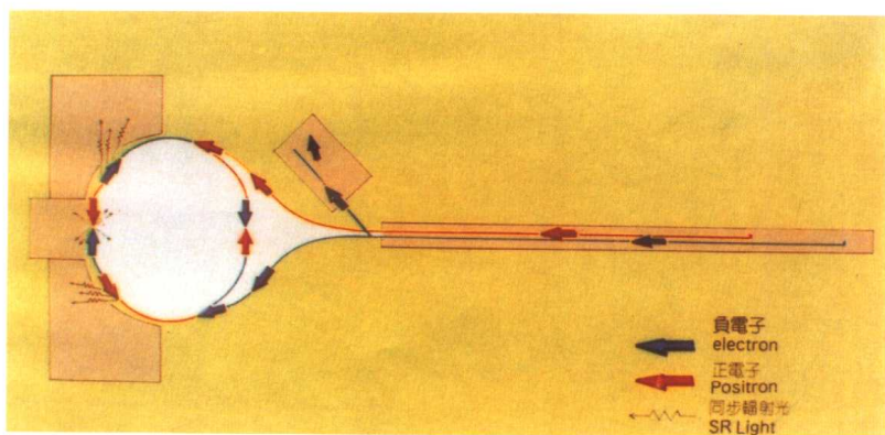
12. 北京正负电子对撞机总体布局和运行示意图
