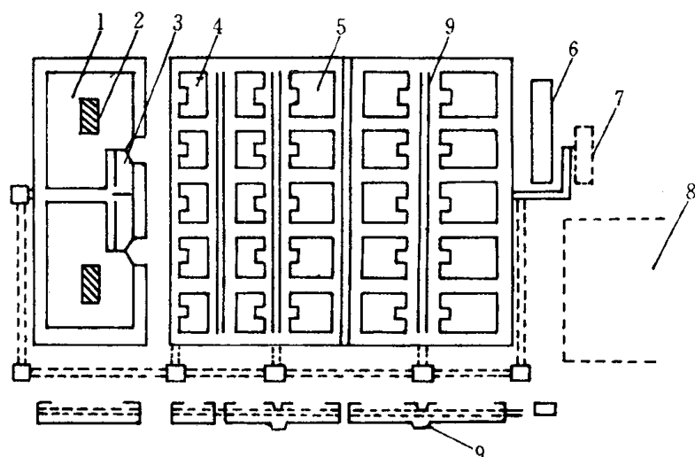
图1 规范化养鳖场的总体布局示意图
