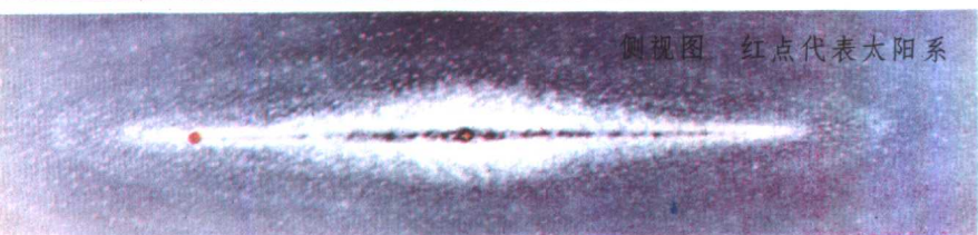
俯视图 十字符号代表银心，三个短黄线条是太阳附近的三条旋臂
