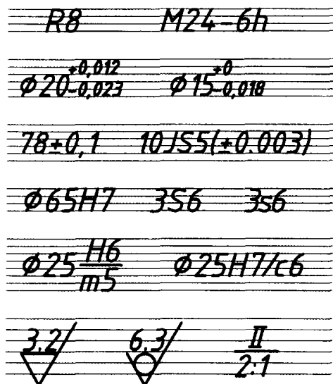
图 1-8 字体综合运用示例
