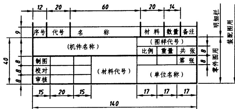
图 1-4 制图作业的标题栏格式及尺寸
