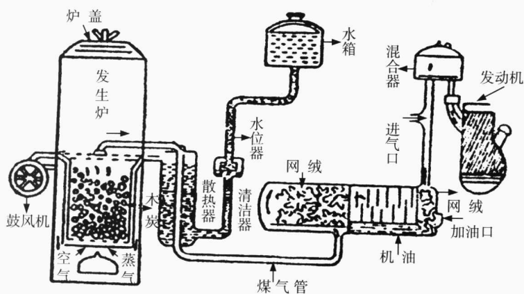
木炭代油炉构造剖面示意图
