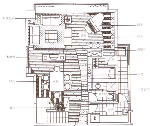
■ 平面图
