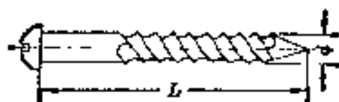
旋入式(单头螺纹)
