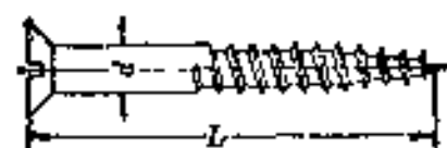
(一字槽)沉头木螺钉 (GB100-76)
