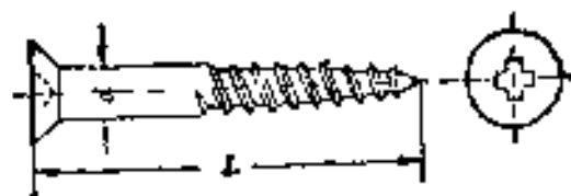
十字槽沉头木螺钉 (GB951-76)
