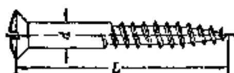
(一字槽)半沉头木螺钉 (GB101-76)
