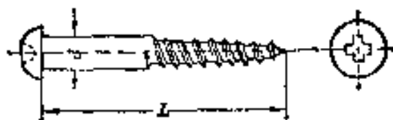
十字槽半圆头木螺钉 (GB950-76)
