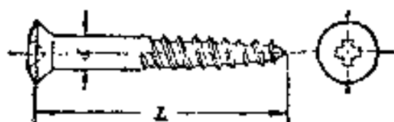
十字槽半沉头木螺钉 (GB952-76)
