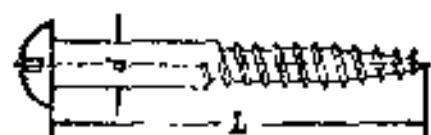
(一字槽)半圆头木螺钉 (GB99-76)
