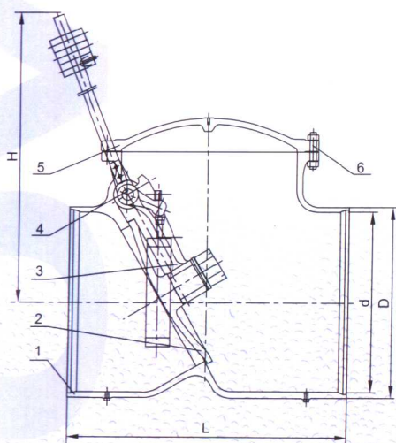
● 抽气止回阀
