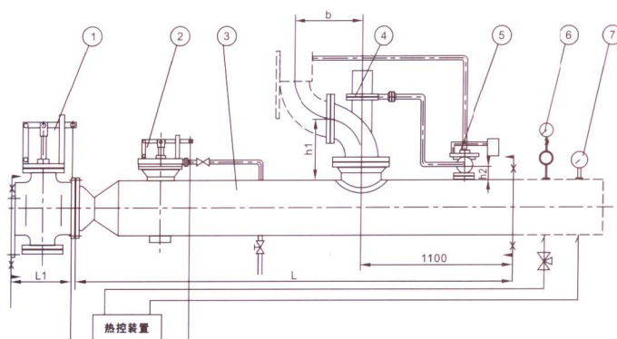
● WY-01 型减温减压装置系列图
