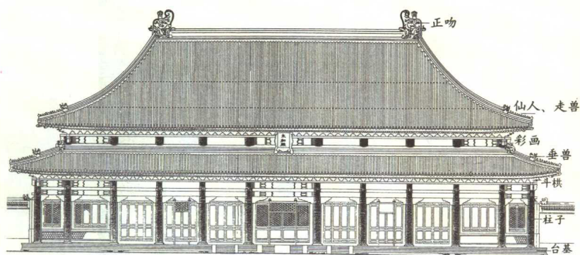
故宫太和殿立面图
