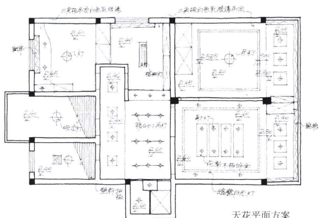
天花平面方案
