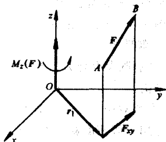
图 2-5 力对轴之矩
