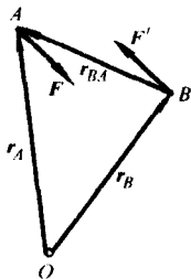
图 2-7 力偶
