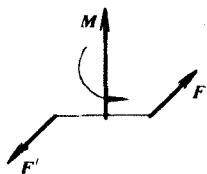
图 2-8 力偶矩矢
