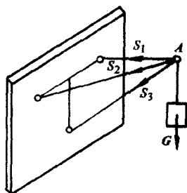
图 2-2 空间汇交力
