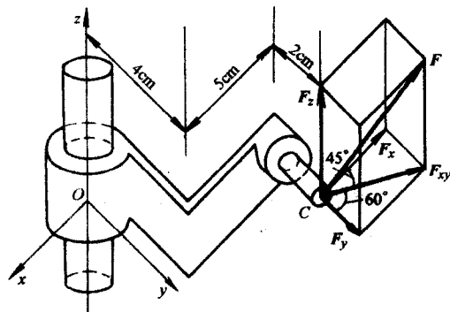
图 2-6 例 2-1 图
