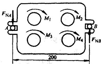
图 2-10 例 2-2 图
