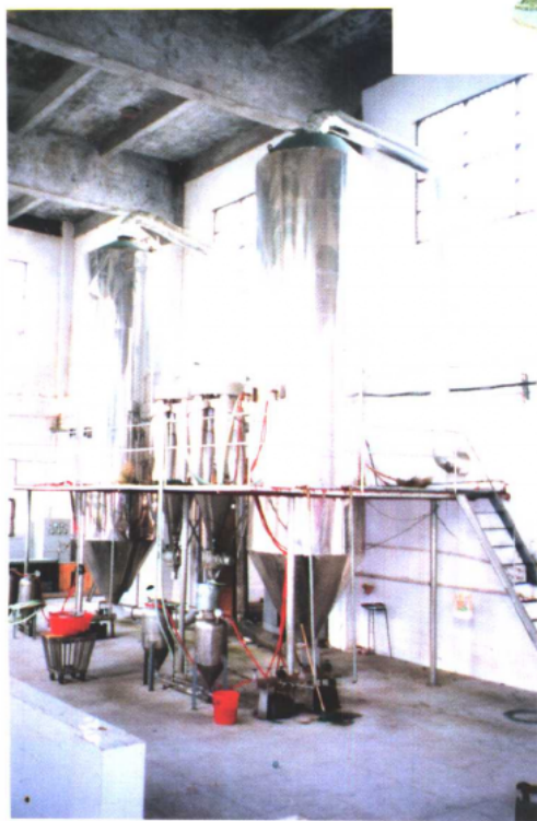
生产粉末油脂用的 压力喷雾造粒设备
