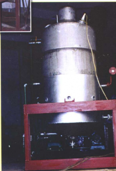
米糠油精炼小型设备
