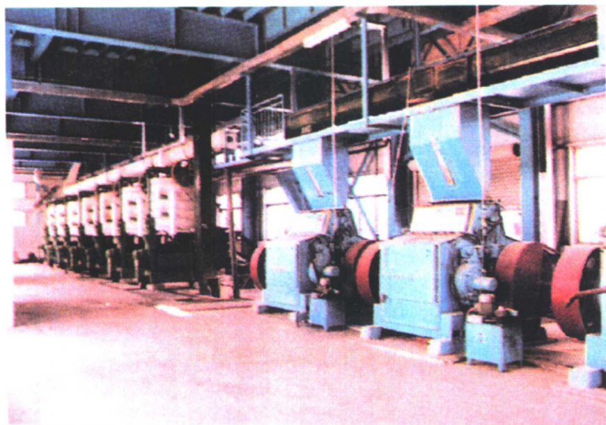
油料预榨车间局部
