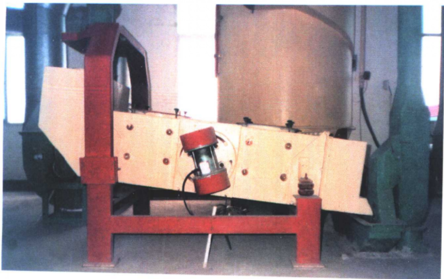
清理油料用的自衡振动筛
