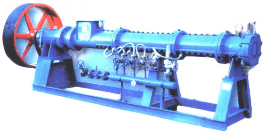
油料预处理用的膨化设备
