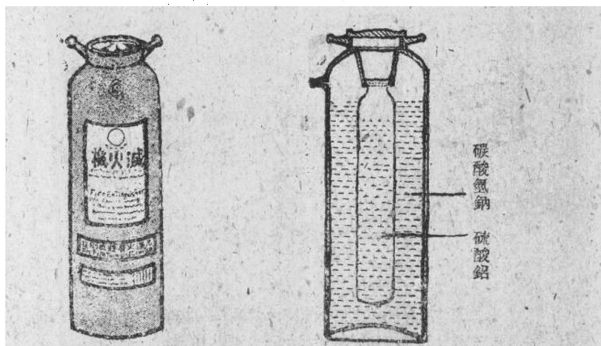
圖 4 化学泡沫灭火器
