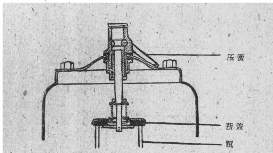
圖8 舟車式泡沫灭火器剖面圖
