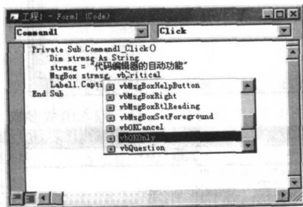
图 1-10 “常数列表”修改函数参数
