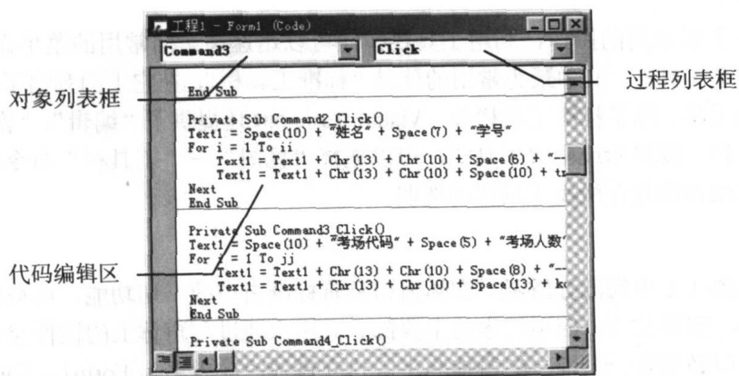
图 1-3 代码窗口
