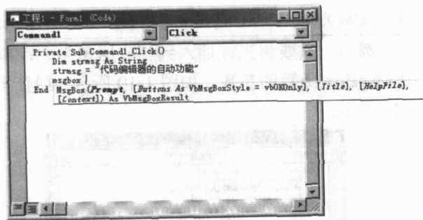
图 1-7 “自动快速信息”输入函数参数
