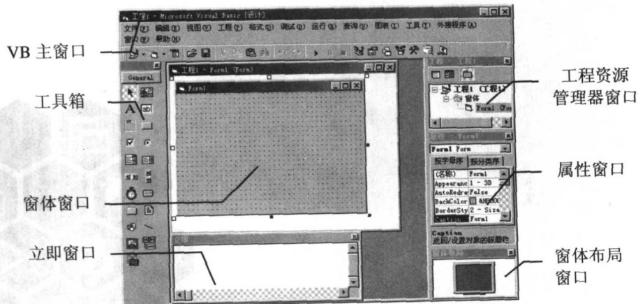
图 1-2 Visual Basic 6.0 应用程序集成开发环境
