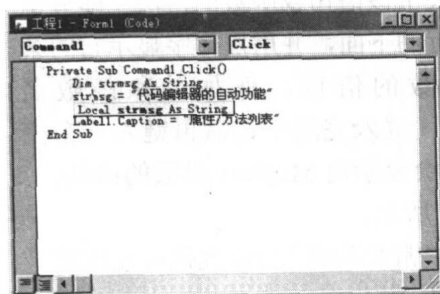
图 1-11 “快速信息”查看变量信息
