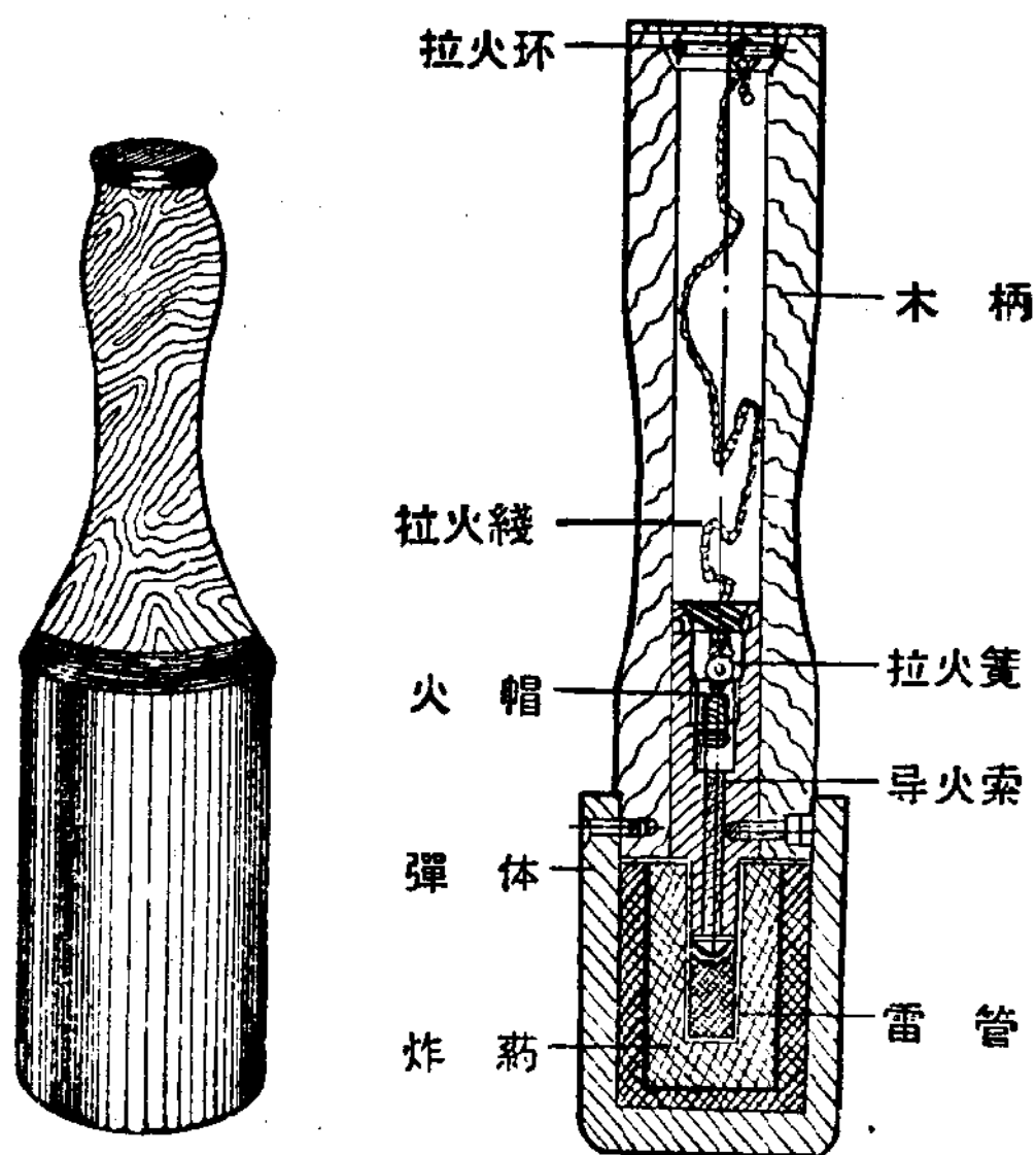
图一 木柄手榴弹构造图
