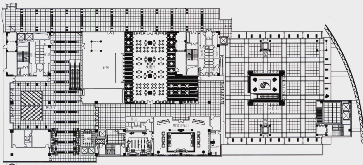
■ 三层平面图
