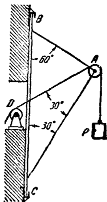
題 27 附圖
