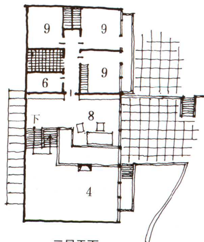
三层平面
