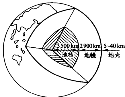
图 1.1 地球的构造
