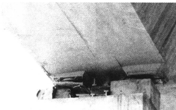
图 1.8 桥梁支座滑移
