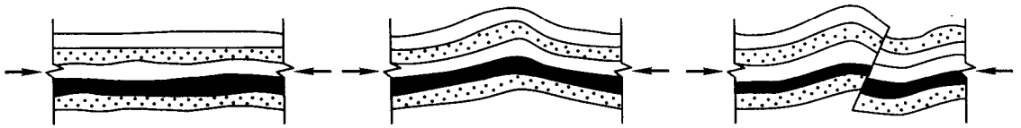
图 1.2 岩层的断裂
