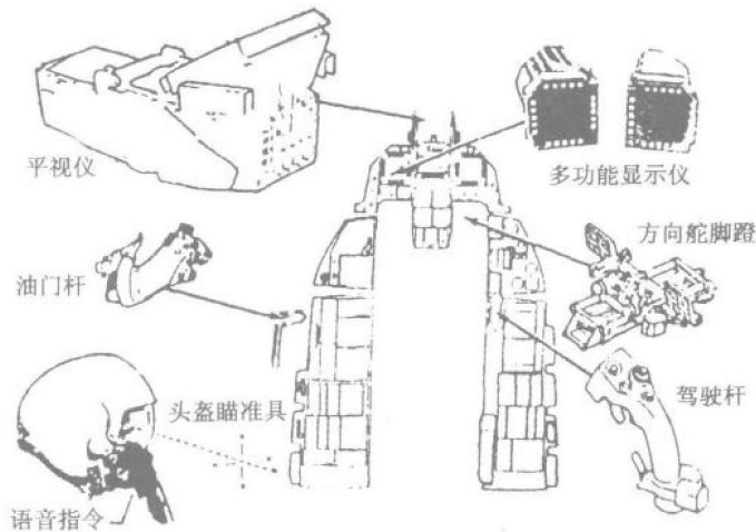
图 1.5 飞机驾驶舱作业域布局示意图
