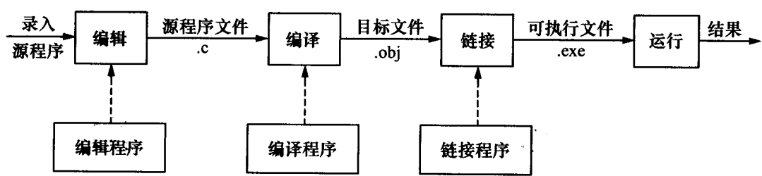
图 1-2 编译执行方式
