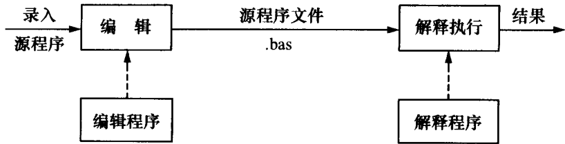
图 1-1 解释执行方式
