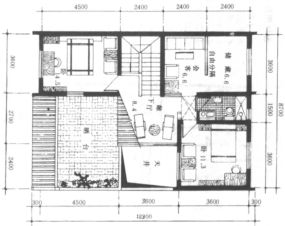
二层平面
