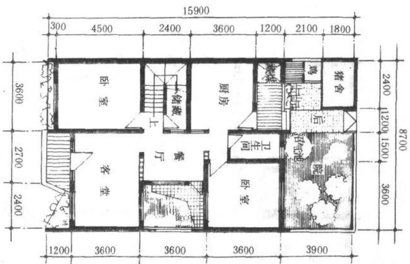
院落平面
