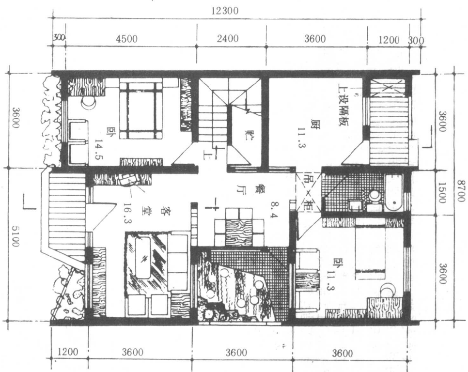
底层平面
