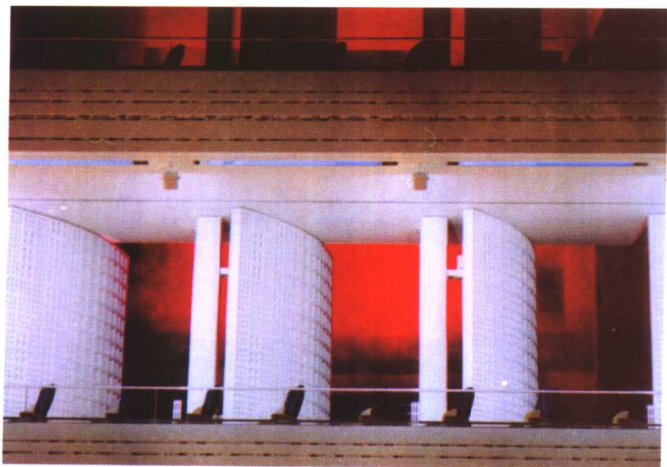
图 41 洛桑音乐厅可调混响室旋转壁面内景
