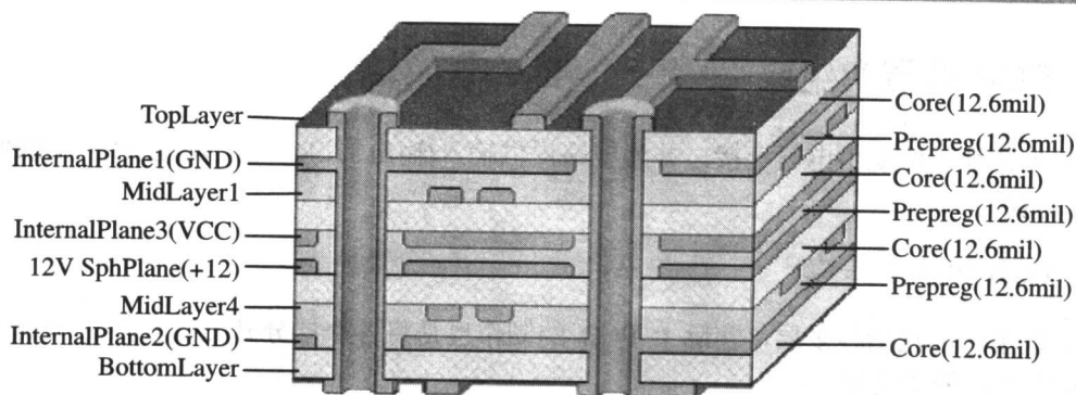
图 1-2 PCB 分层和组成示例
