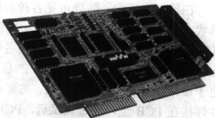
图 1-1 PCB 的外观
