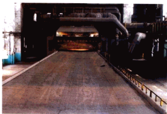
△ 二炼铁厂 265 米 2 烧结机
