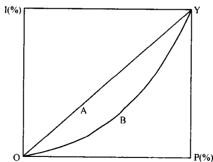
图 1-1 洛伦茨曲线示意图
