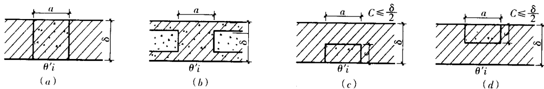
图 2-1 热桥形式
