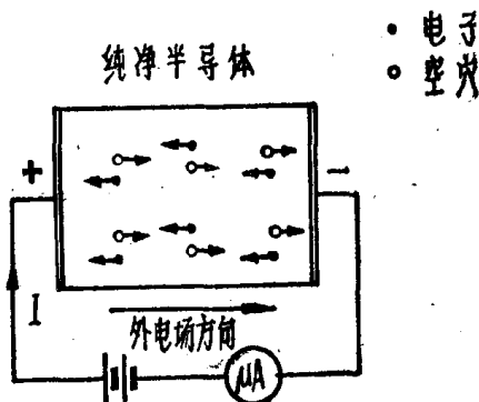
图 1-4 半导体中的电流等于电子流和空穴流之和
