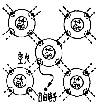
图 1-3 本征激发产生的电子——空穴对
