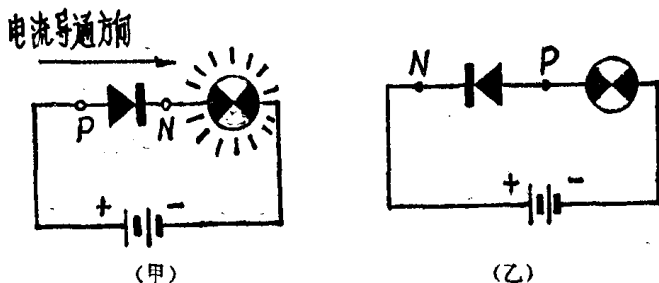
图 1-8 PN 结单向导电实验
