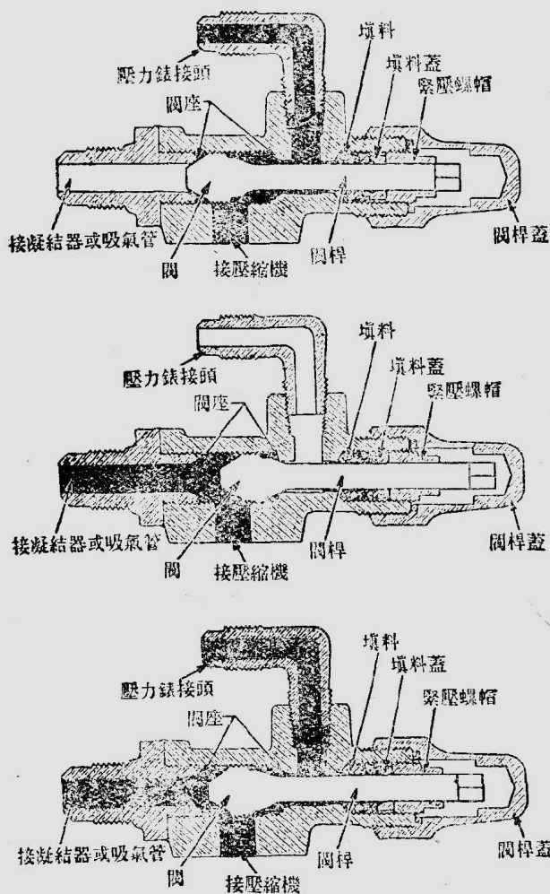
圖 4. 裝在壓縮機非吸氣二邊的修理閥, 在三種不同位置上的情形。
