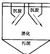
图 1-8 Imhoff 池
