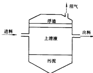
图 1-9 传统消化池
