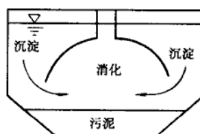
图 1-7 Travis 池
