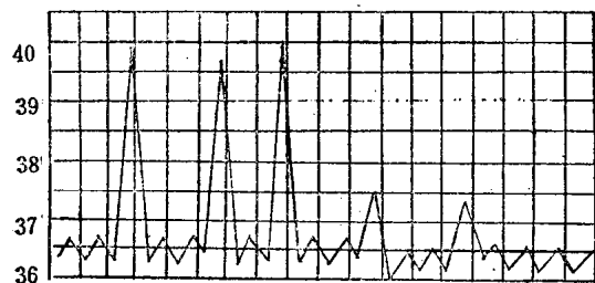
图 2-3 间歇热
