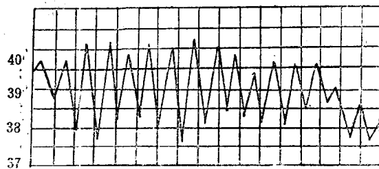
图 2-2 弛张热
