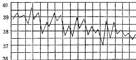
图 2-4 不规则热
