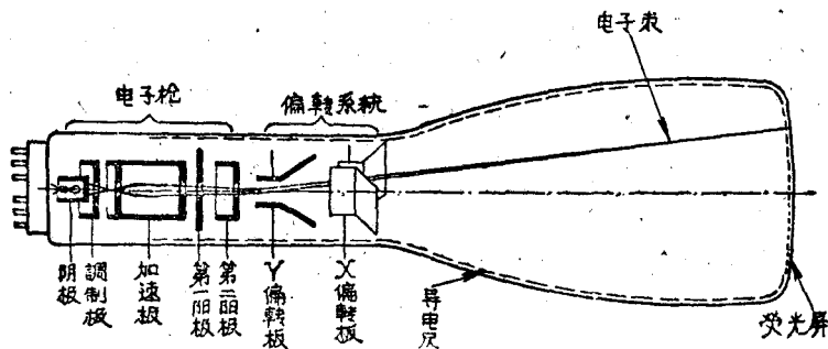
图(1.1) 电子束管的典型結構。
