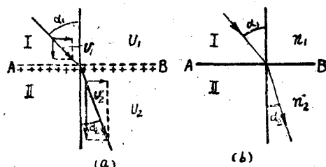
图(2.1) 电子束在偶电层上的折射。
