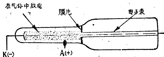
图(1.2) 勃朗管。
