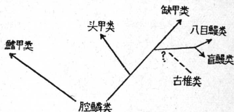
图5 无颌类的系統发生图(依尼柯里斯基)
