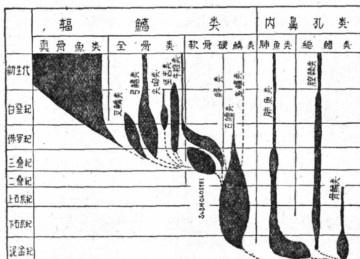
图 14 硬骨魚类演化图
