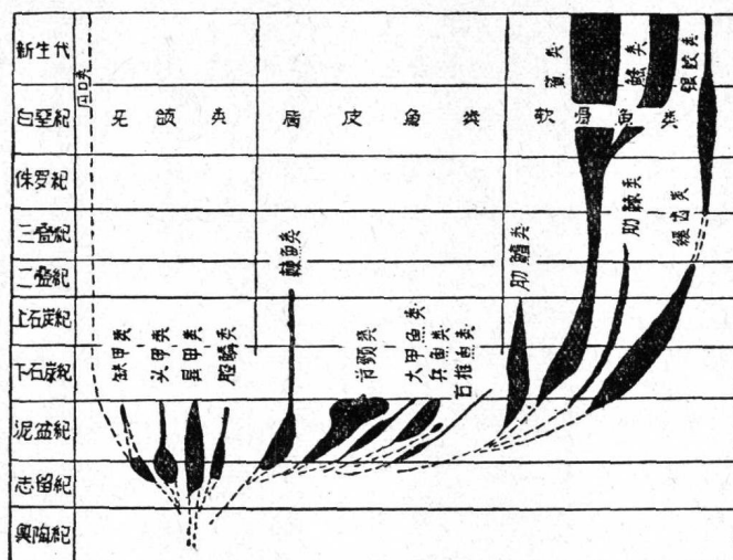
图 11 无颌类、盾皮类及软骨鱼类的演化
