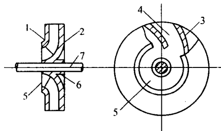
图 2.5 单吸式叶轮
