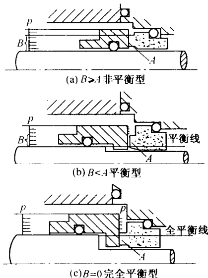
图 2.11 平衡型和非平衡型机械密封
