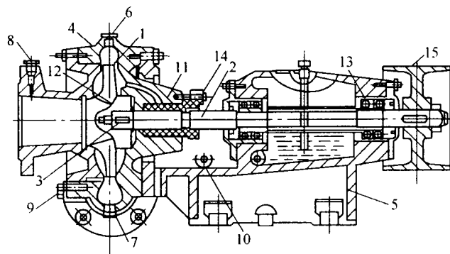
图 2.4 单级单吸卧式离心泵
