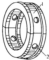
图 2.9 水封环
