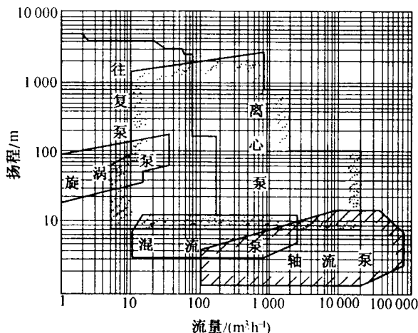
图 1.3 常用的几种水泵总型谱图
