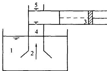
图 1.2 容积式水泵的工作原理
