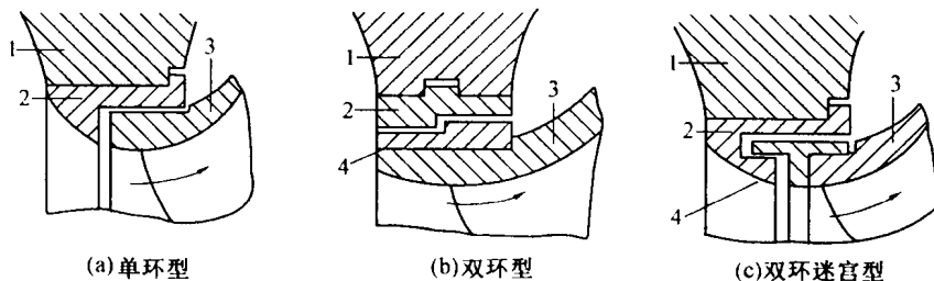
图 2.12 减漏环
