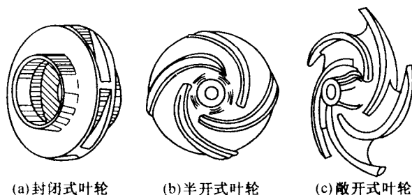
图 2.7 叶轮形式
