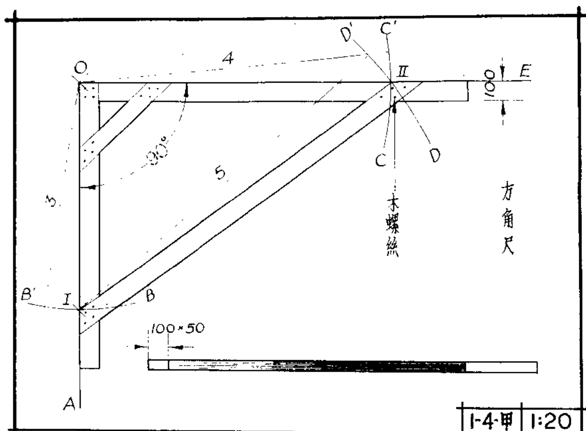
用方角尺兜方法
