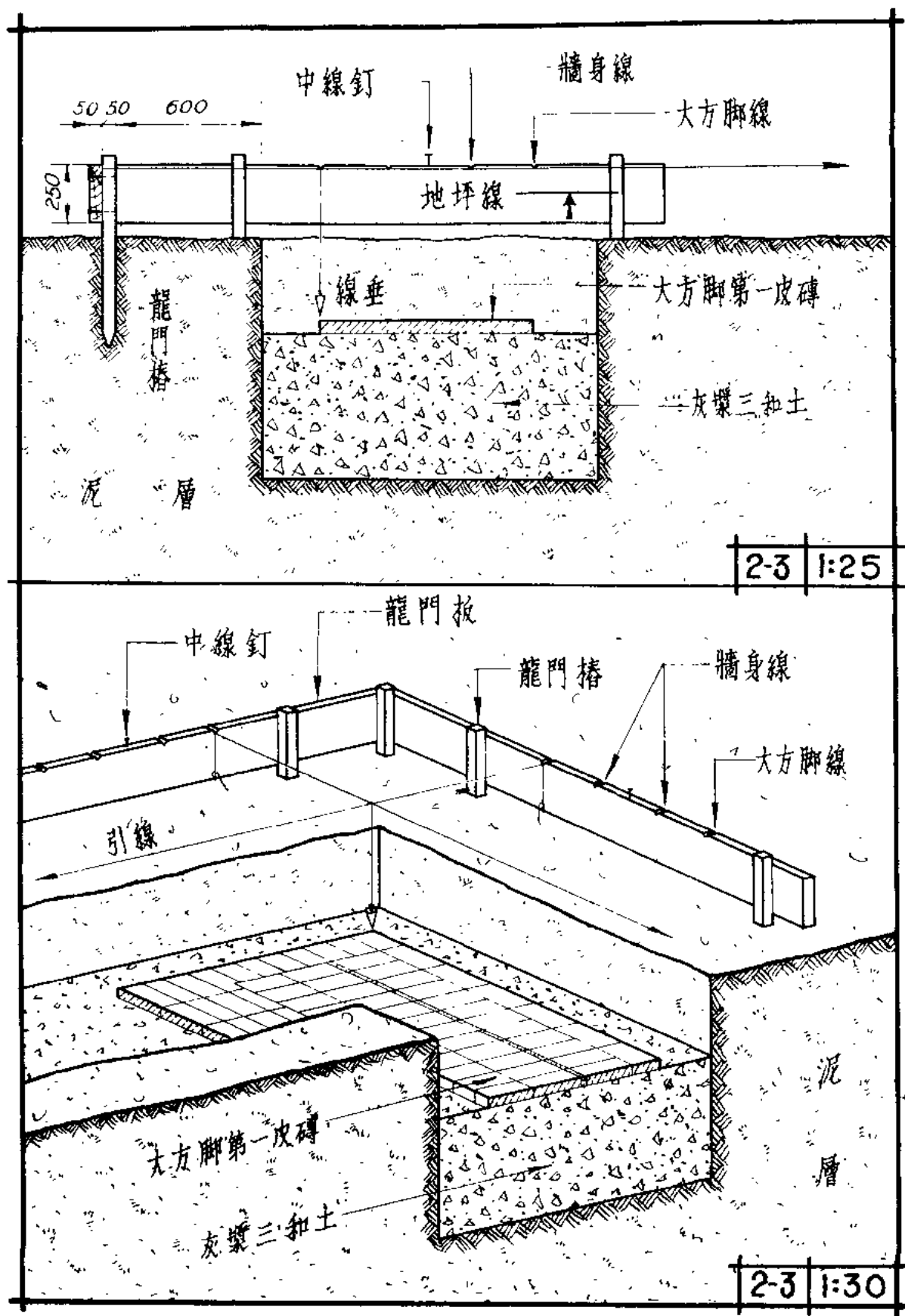
圖2-3. 大方腳位置引線詳圖
