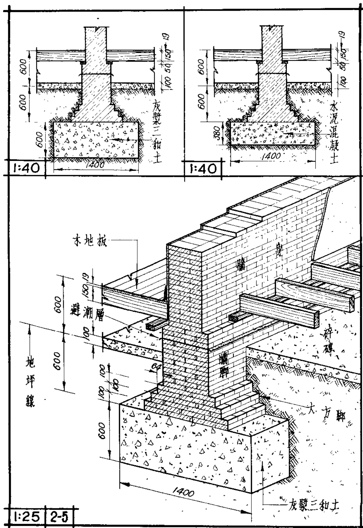
圖 2-5. 一磚半厚牆, 牆基疊砌詳圖
