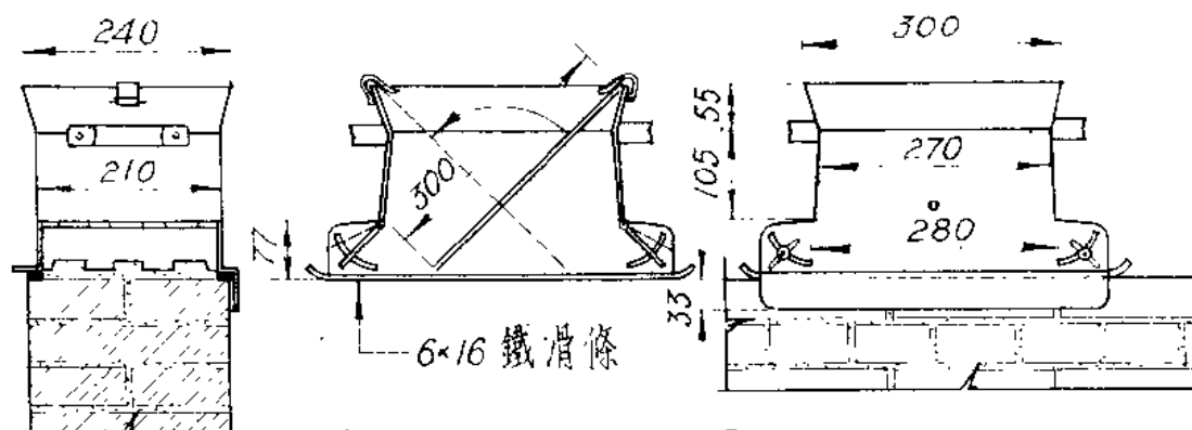
鋪灰器
