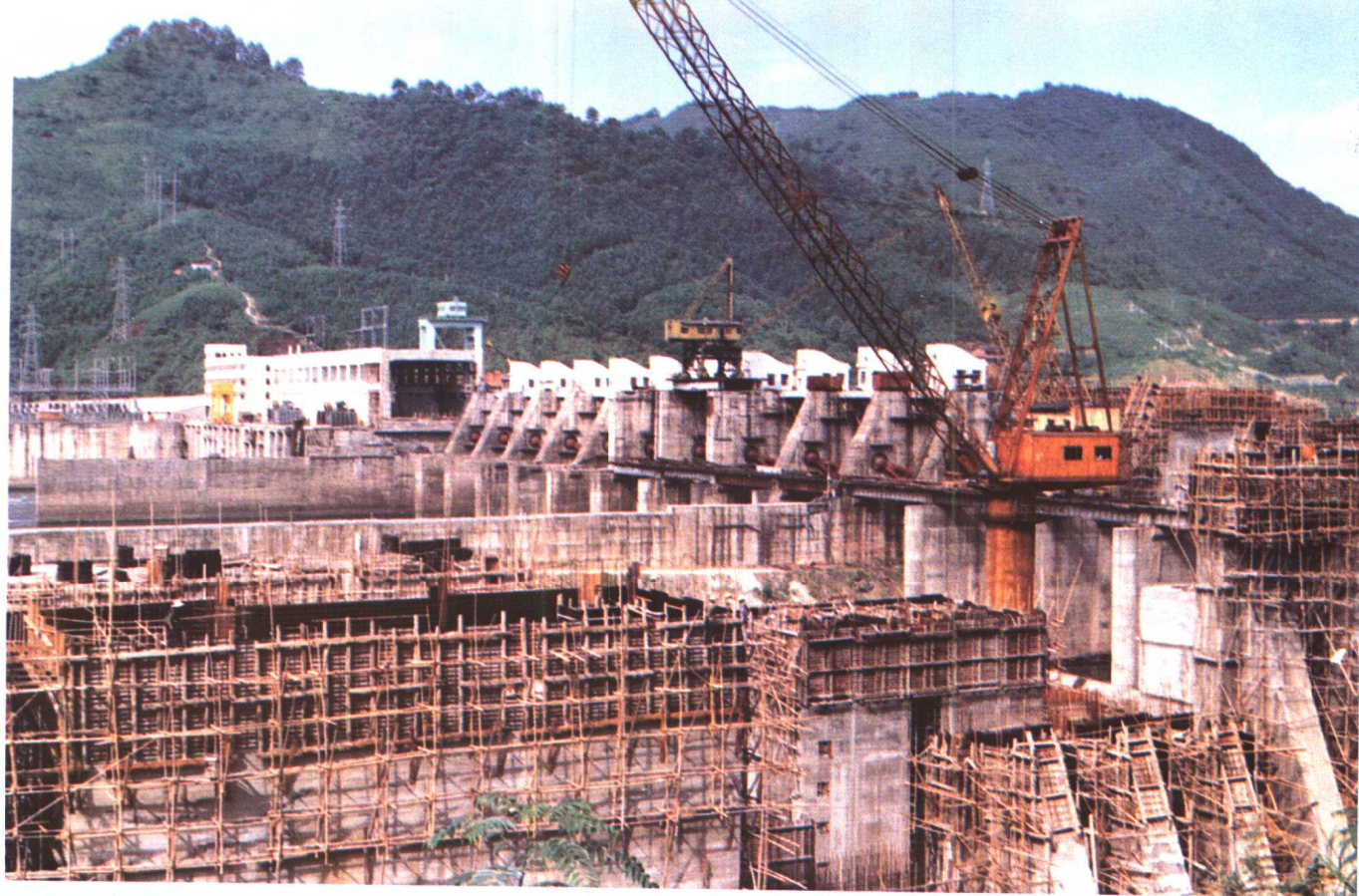
国家重点工程——沙溪口水电站三台7.5万千瓦机组已投产，4号机组正在安装中。 (林辉龙 摄)
