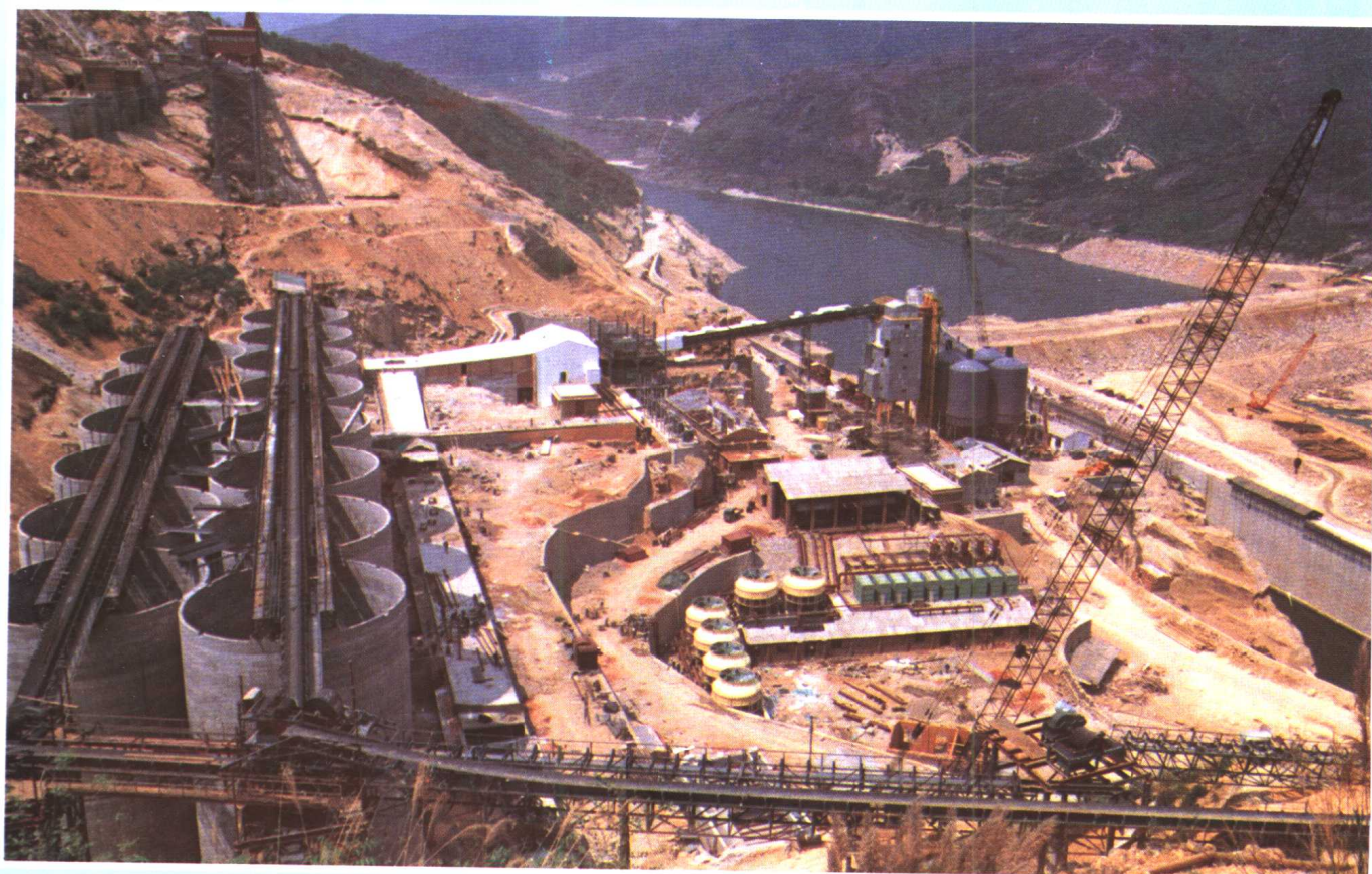
国家重点工程——福建水口电站上游主围堰已筑高40余米，达防洪高程，明溪导流已完工，电站基础设施及附属工程正加紧建设，整个工程已具雏形。 (林辉龙 摄)
