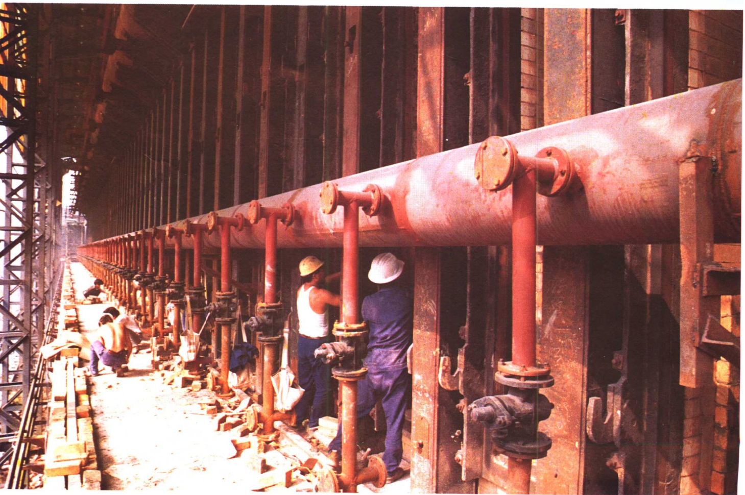
三明钢铁厂年产50万吨钢的重要配套工程——65孔焦炉经过三年紧张施工，于1990年9月投产。
