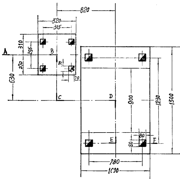
ABCDEF 剖面
