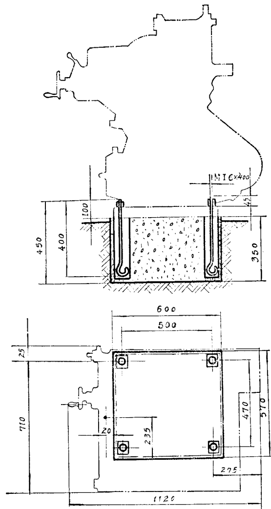
安装基础图
