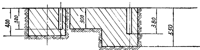
ABCDEF 剖面
