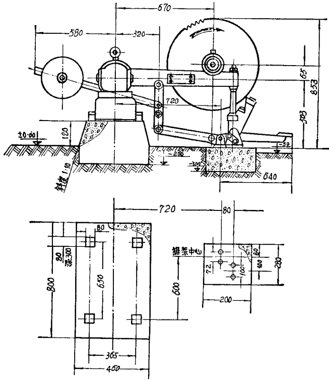
安装基础图
