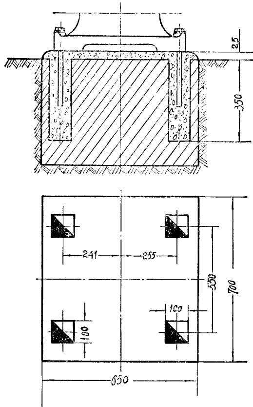
安 装 基 础 图
