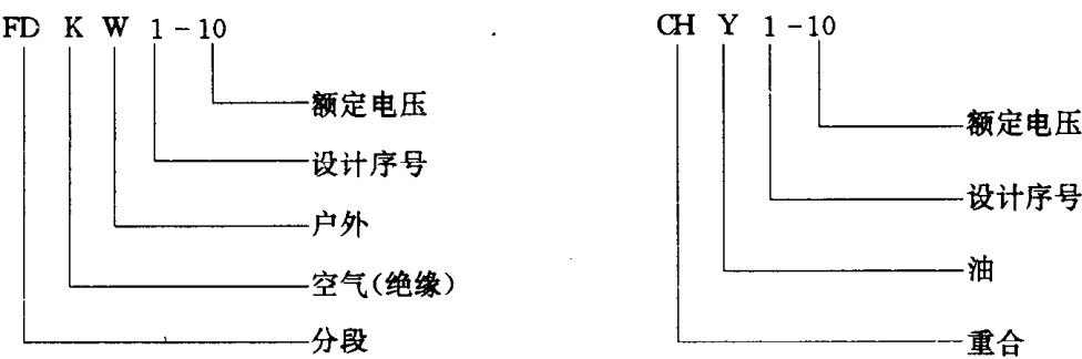
分段器
