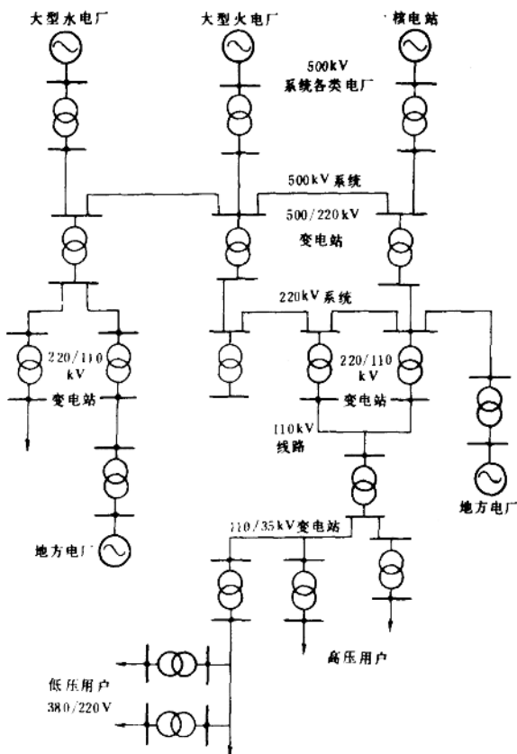
图 1-1 电力系统基本构成
