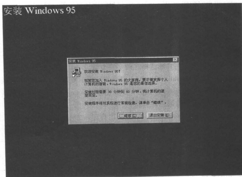
图 1.1 Windows 95 的安装
