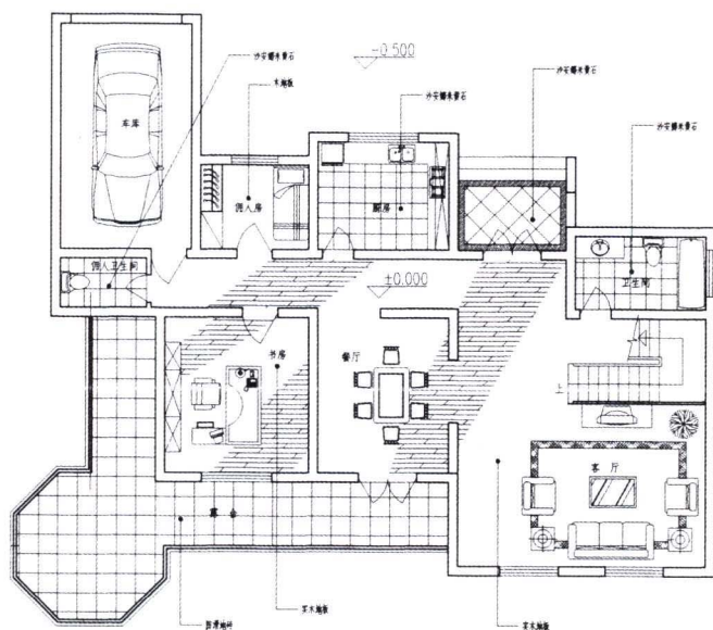
别墅1层平面图
