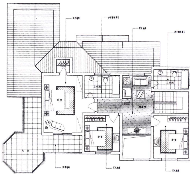
别墅2层平面图
