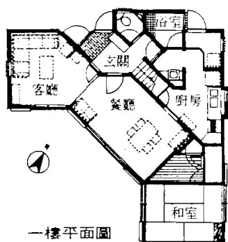
一樓平面圖
