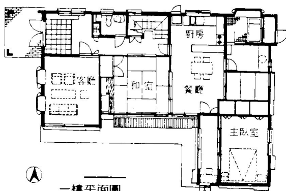
一樓平面圖
