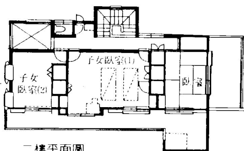
二樓平面圖
