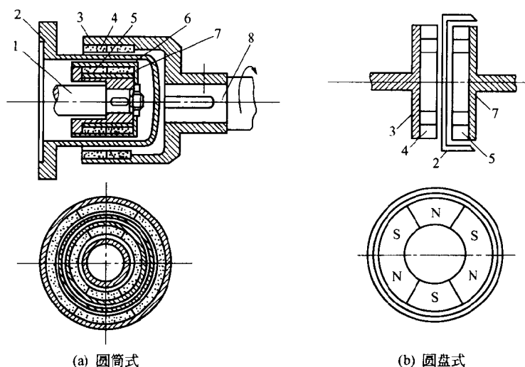
图 1-1 磁力驱动器结构示意图
