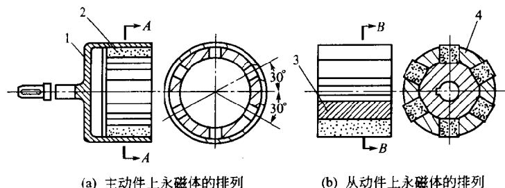
图 1-2 间隙分散式永磁体在磁筒上的排列
