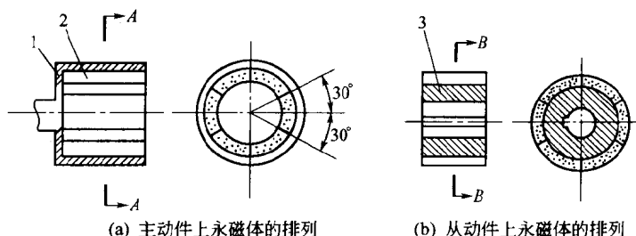
图 1-3 组合拉推式永磁体在磁筒上的排列
