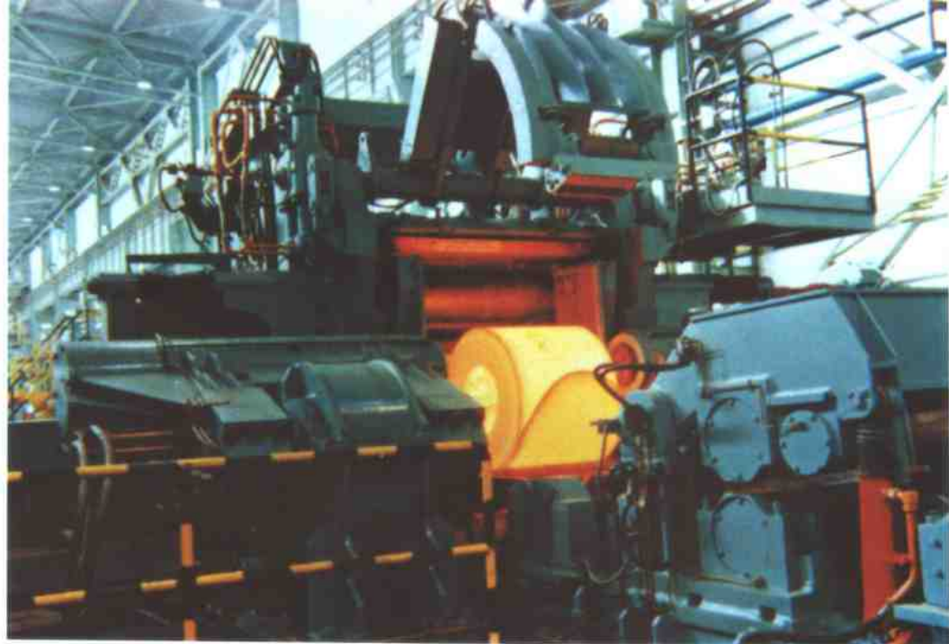
从加拿大引进的我国第一台热卷箱
