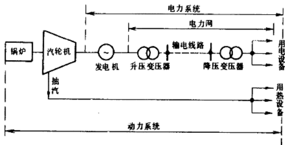
图 1-1 动力系统、电力系统及电力网示意图
